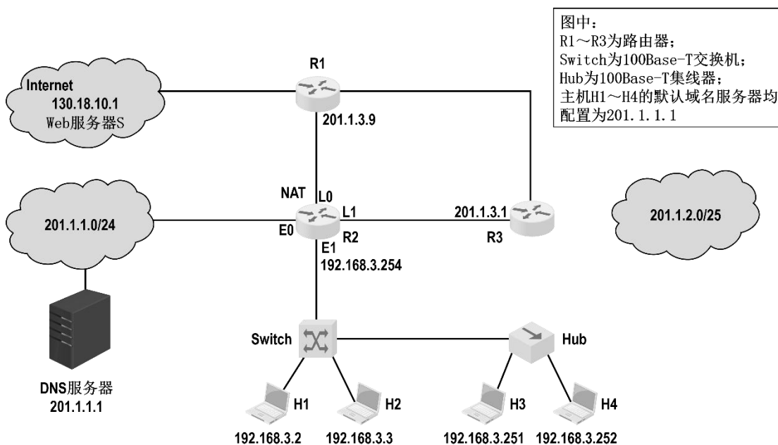
图 6-53 习题 6-36 的图
